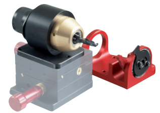
Schleifeinrichtung für Stufenbohrer inkl. 1 Spannfutter Drm. 3,0 - 12,0 mm (erfordert Kreuztisch Art.-Nr.: 48007)
